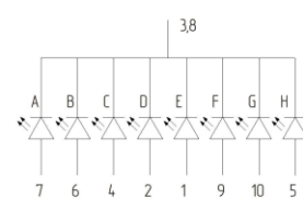
ИПЦ57А1-1/7
