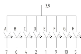
ИПЦ57А-1/7
