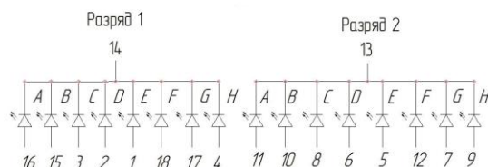
ИПЦ57А1-2/7
