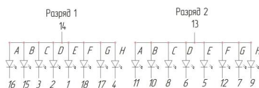
ИПЦ57А-2/7
